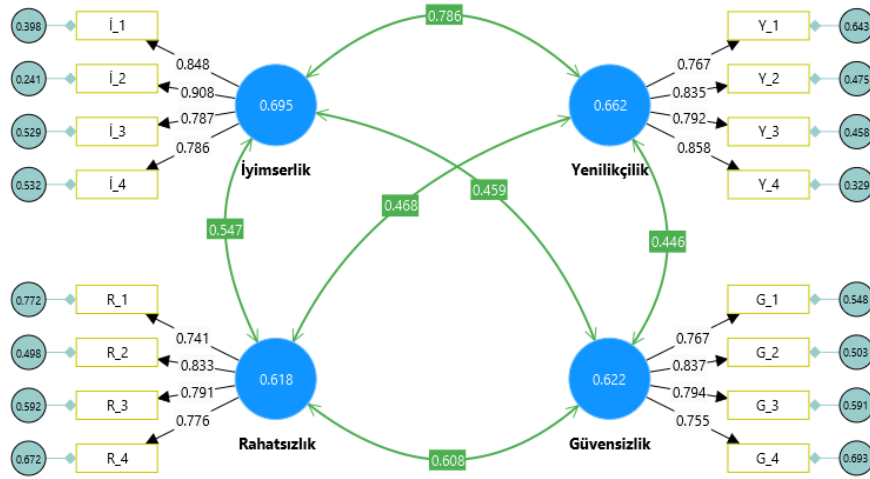
Şekil 3: Reflektif Birinci Düzey Yapı DFA Sonuçları
